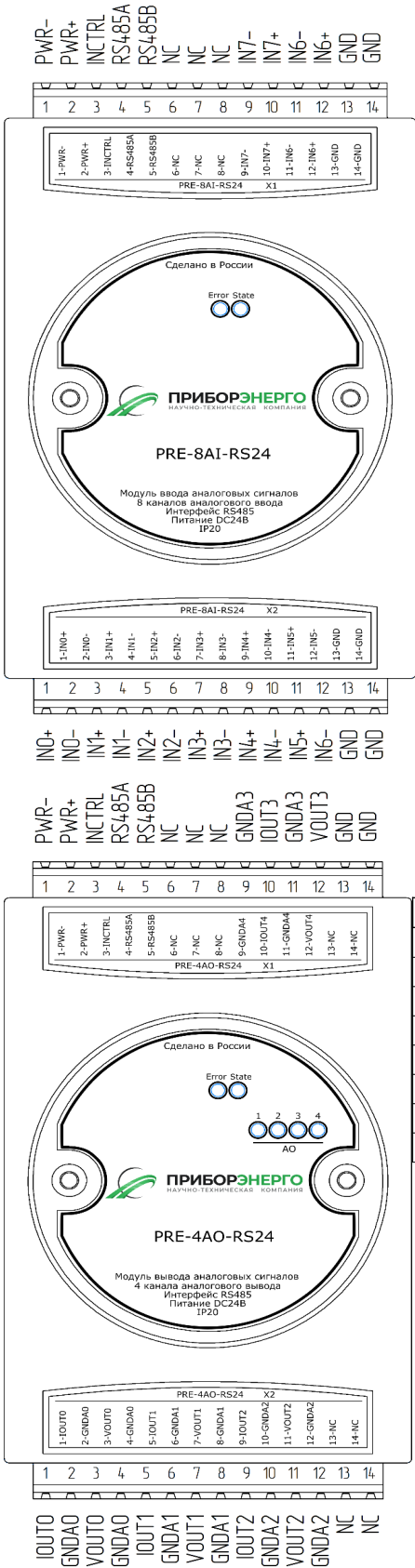
Рис. 1. Внешний вид и схема подключения модулей серии PRE-xAI и PRE-xAO
