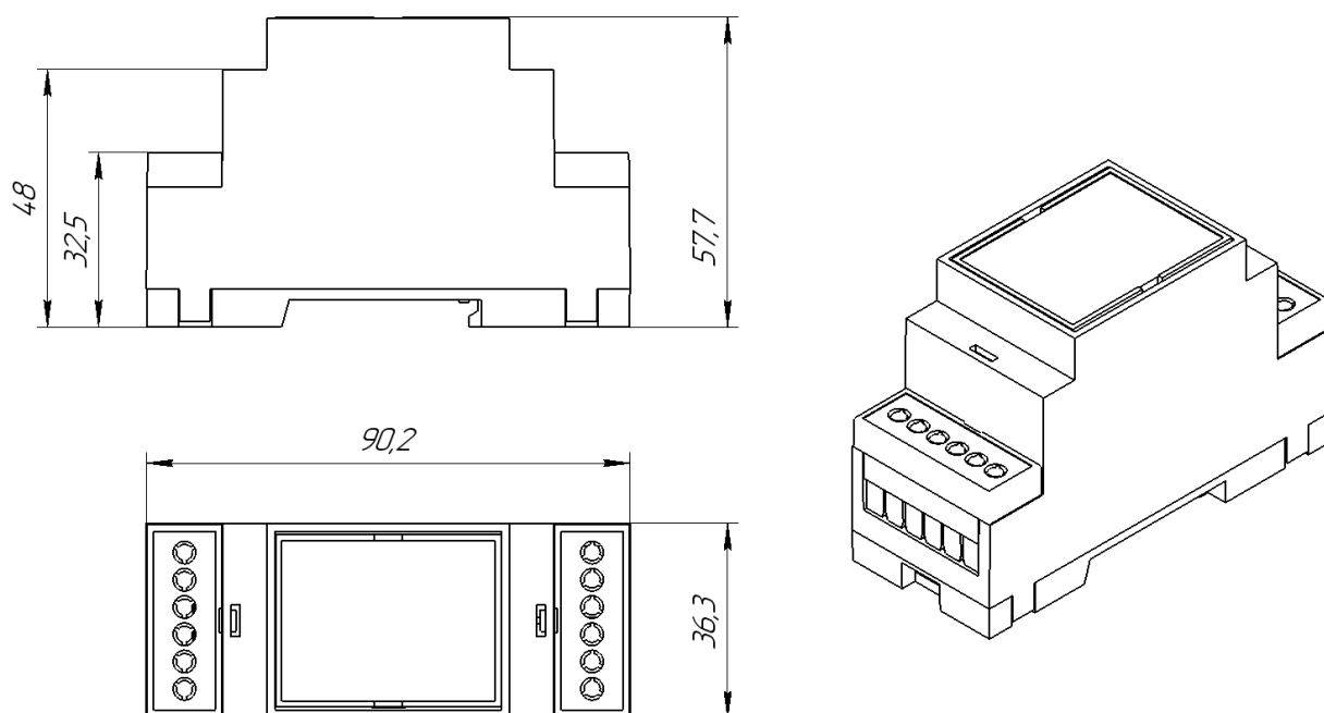
Рис. 1. Внешние размеры БП
