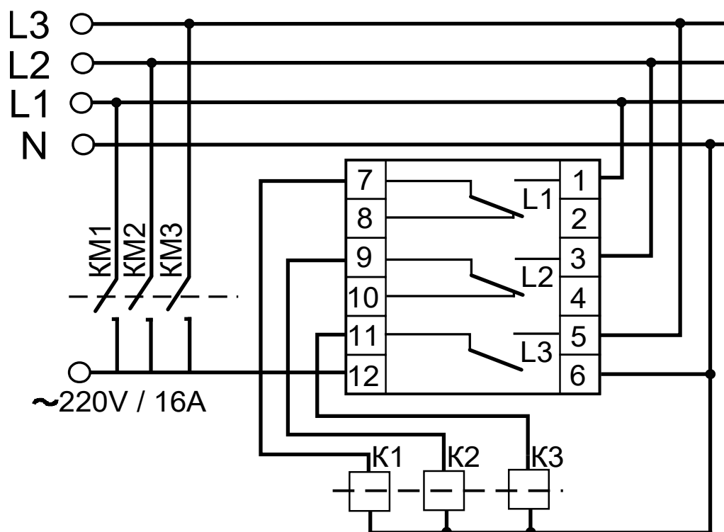
Рис.3. Схема подключения ПЭФ-301 при величине нагрузки более 16А с использованием магнитных пускателей
