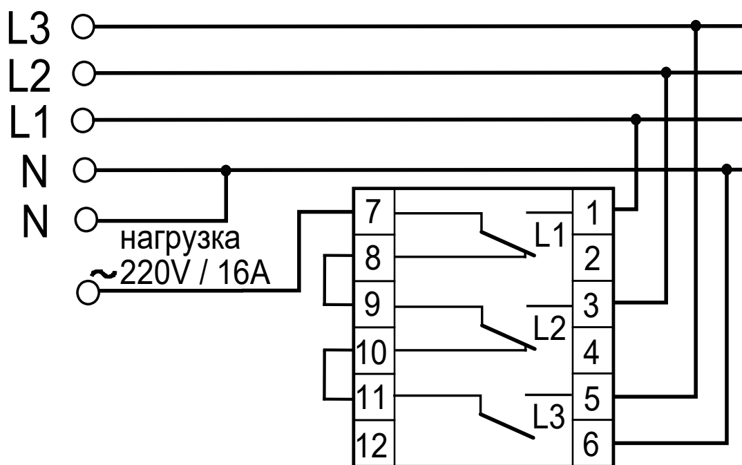
Рис.2. Схема подключения ПЭФ-301 при величине нагрузки до 16А
