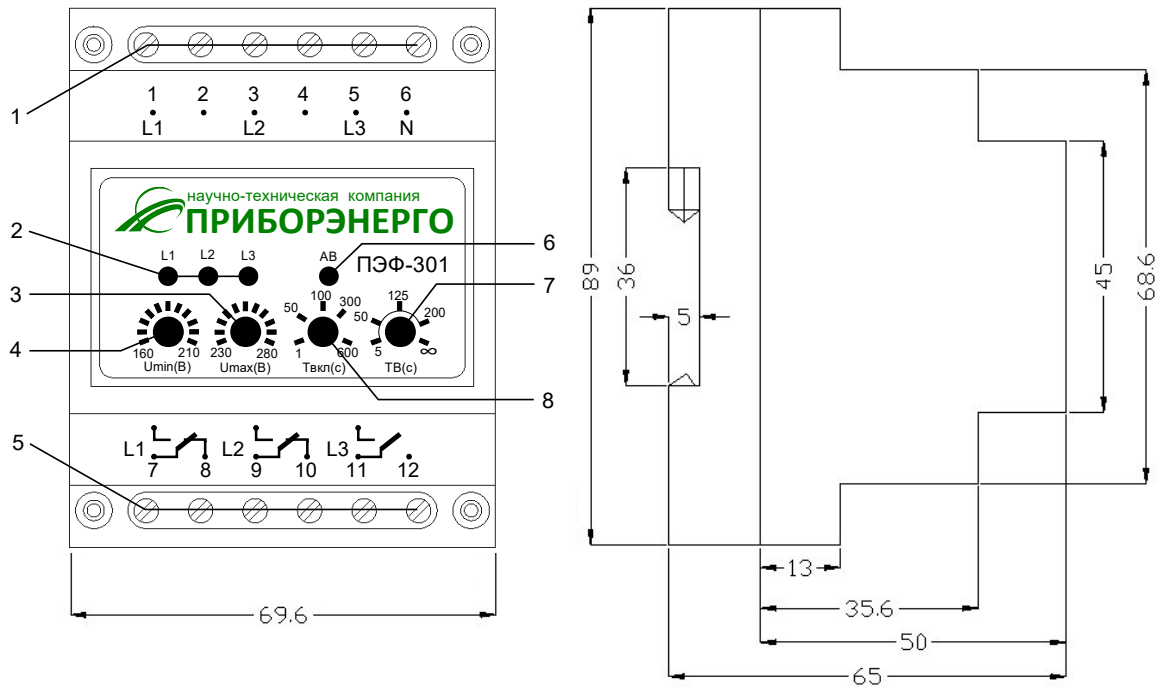
Рис.1. Внешний вид и габаритные размеры
