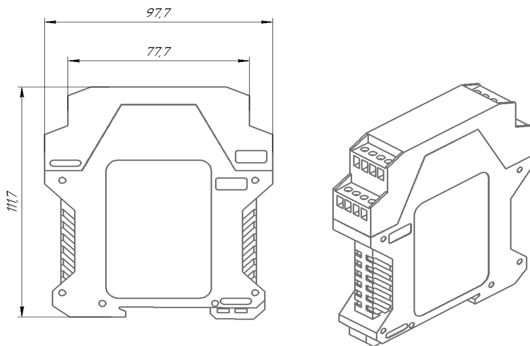
Рисунок П4. Габаритные размеры реле «РКТУ-1» (конструктив на DIN рейку)
